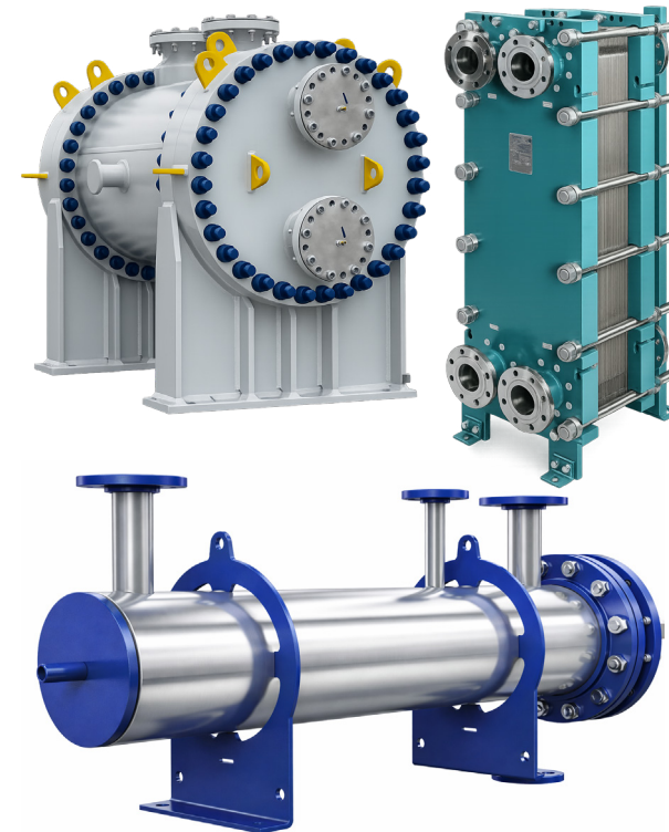
Intercambiadores de calor -Carcasa y tubo -Carcasa y placas -Tipo Placas
